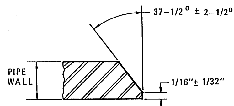
WELDING BEVEL EDGE
